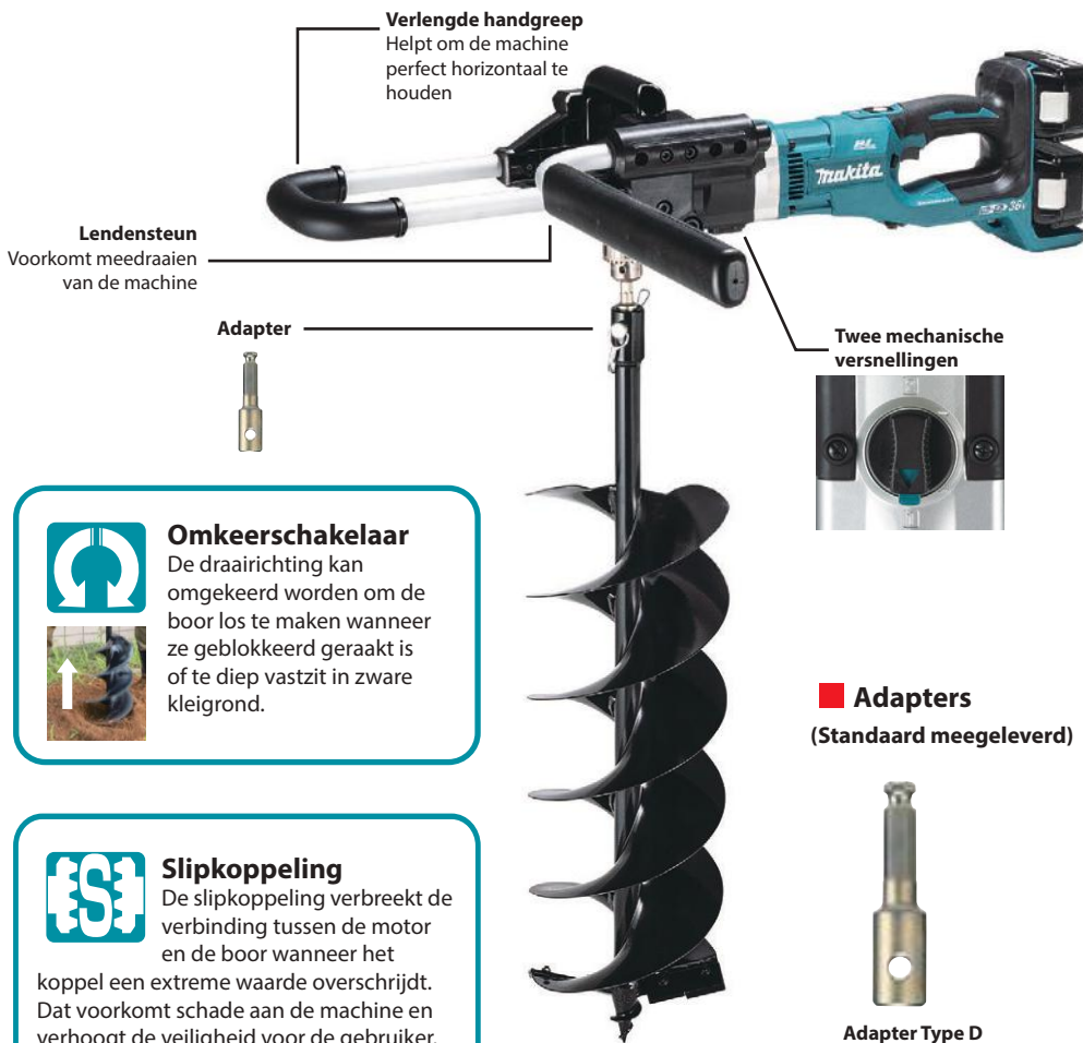
Adapter Type D voor Makita-grondboren Ref. 327687-6
